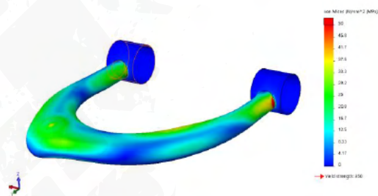
Max Von Mises Stress = 50 MPa
