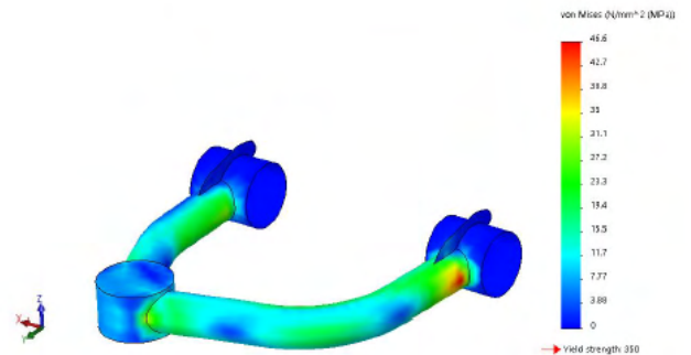
Max Von Mises Stress = 46.5 MPa
